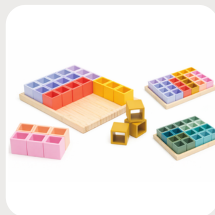
Rompecabezas geométrico
